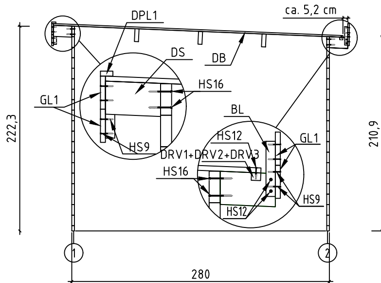
Cross section - Schnitt - Vu de coupe - Sezione trasversale - Doorsnede - Lõige A - A
